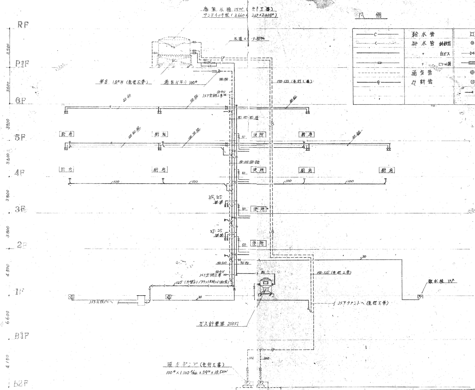
配管系統図 NO scale
