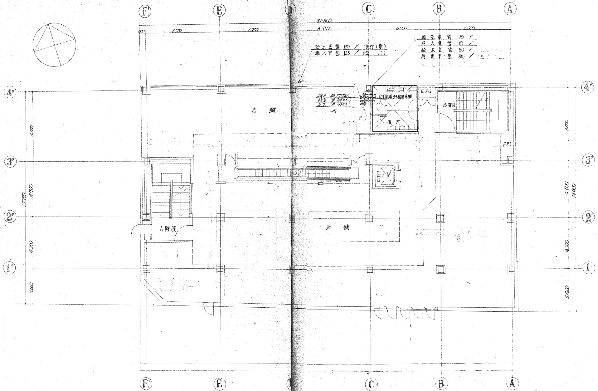
3階平面図
