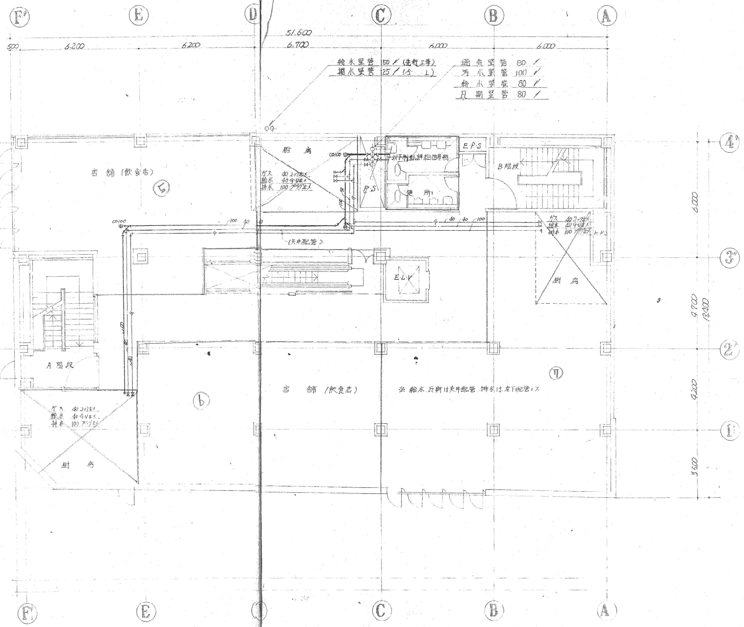
5階平面図
