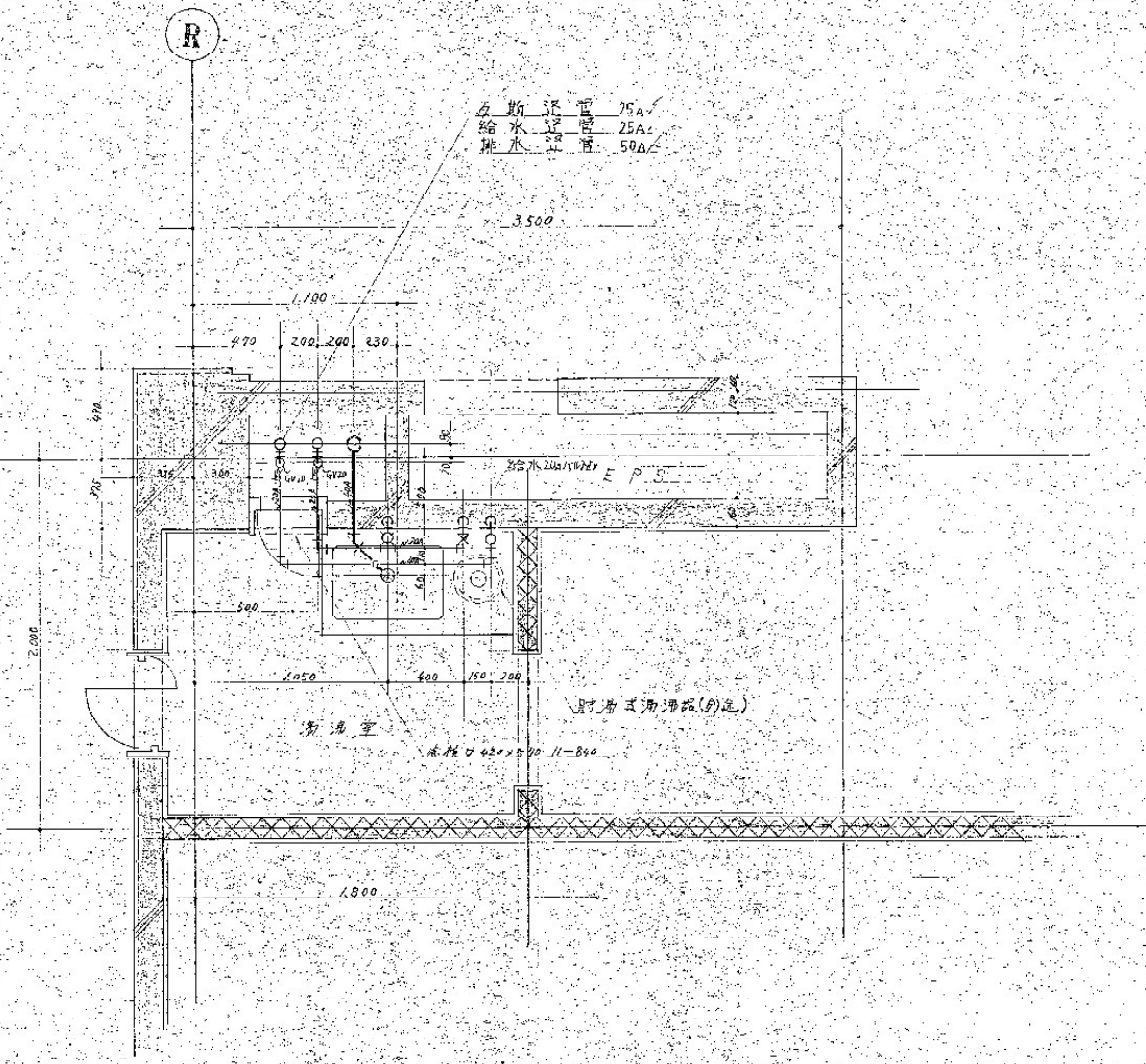
3~5階浴室詳細図 1/20
