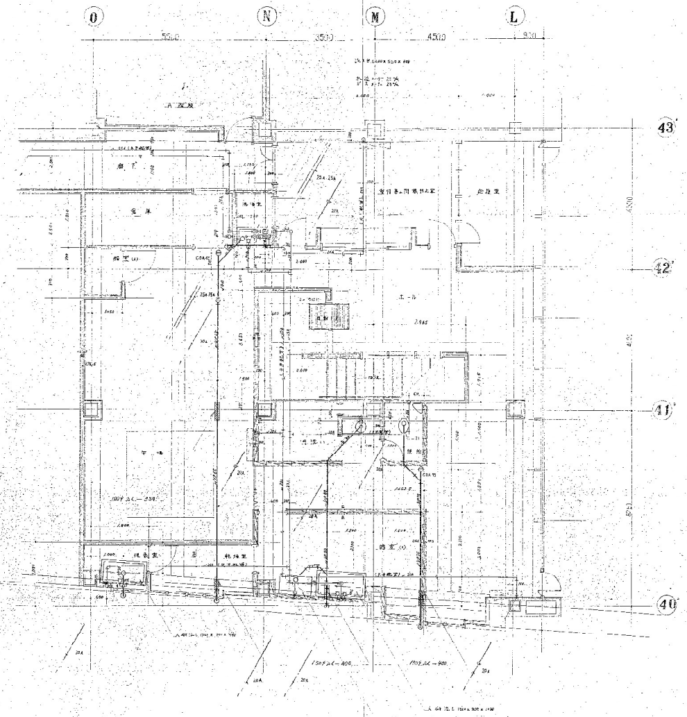
新田平尾路平面図 1/50 凡例 1. 1500 x 400 2. 給気口 3. 採光口 4. 採光口 5. 採光口
