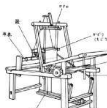
機織機（トントカラ）
