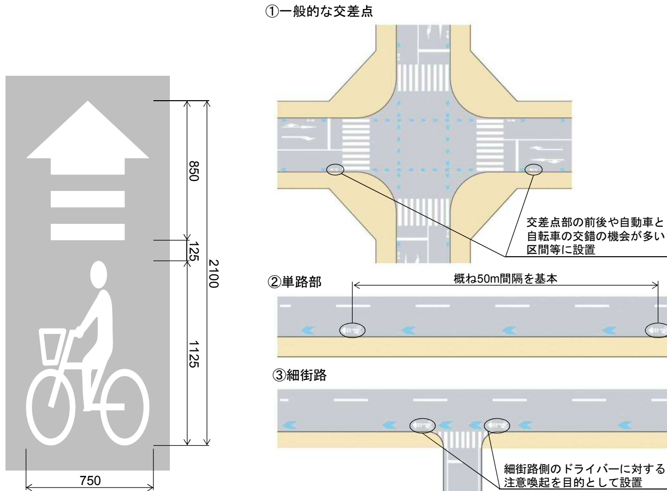
図5-2. 自転車のピクトグラム
