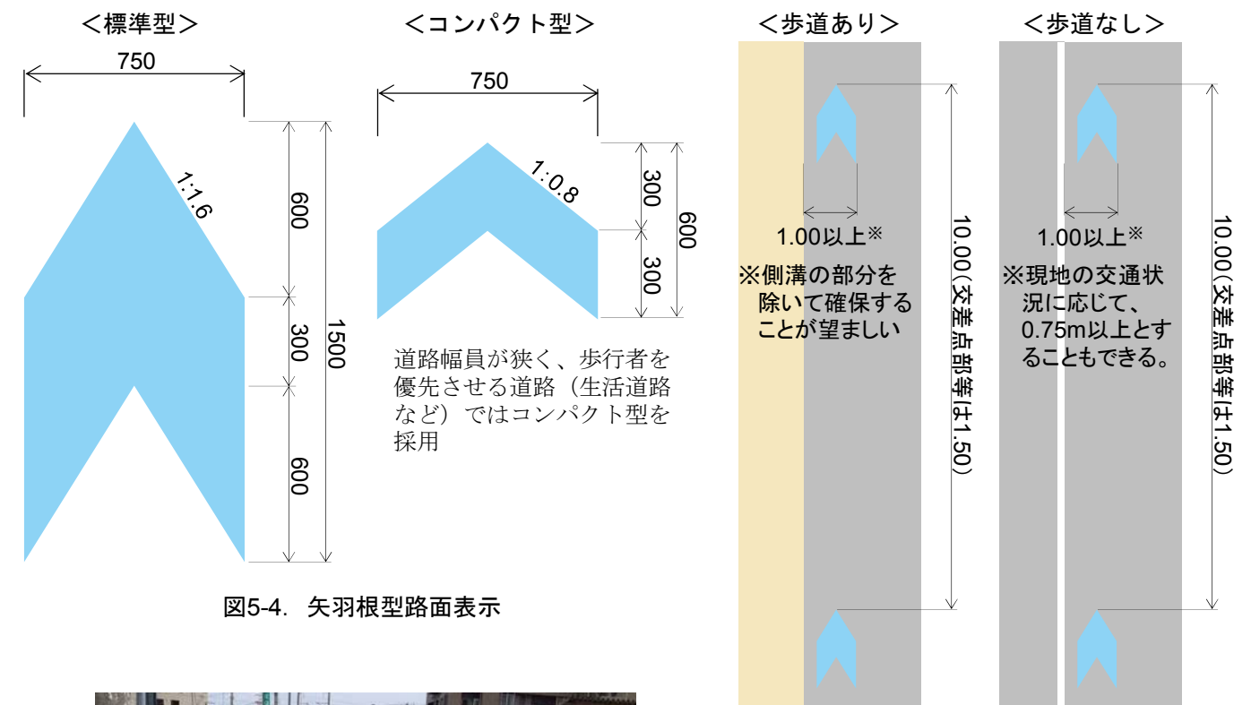
図5-5. 矢羽根型路面表示の設置位置
