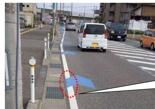
図5-6. 矢羽根型路面表示と外側線が重なる場合
