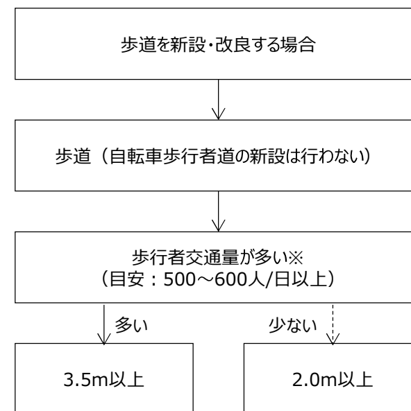
図3-2. 歩道・自転車歩行者道の考え方
