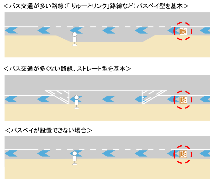
図5-9. バス停注意のピクトグラムの設置位置
