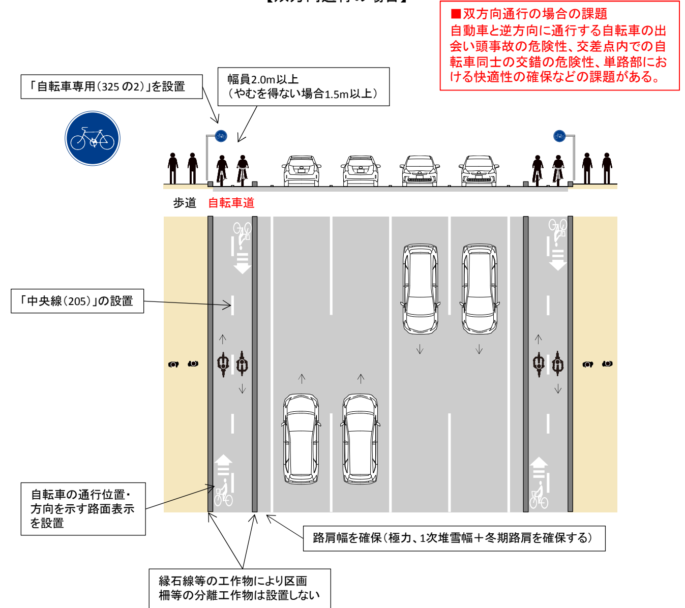
【双方向通行の場合】
